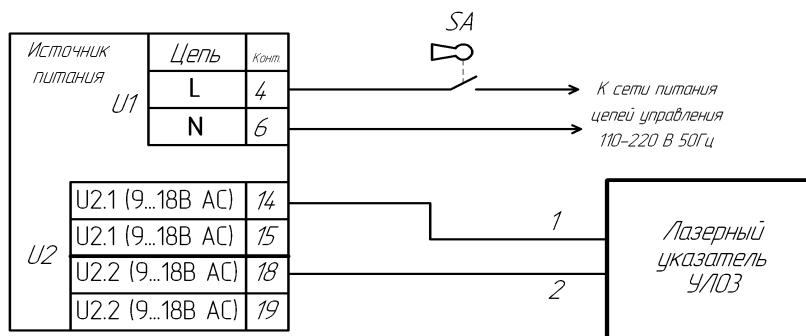
Рисунок 4. Схема подключения лазерного указателя к цепям 110-220В 50 Гц с внешним источником питания.
